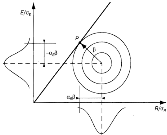
Рис. 2. Характеристика безопасности в плоскости безразмерных переменные E / \sigma_E , R / \sigma_R
