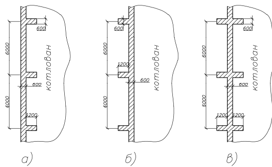
Рис. 4. Схеми влаштування контрфорсів в поздовжній стіні котловану:
